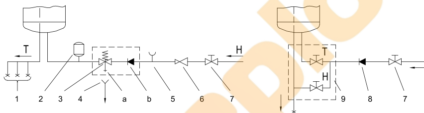
Напірна (закрита) система
